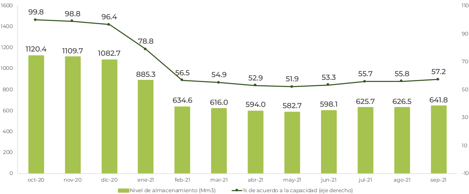
NIVEL DE ALMACENAMIENTO DE AGUA Y PORCENTAJE RESPECTO A LA CAPACIDAD DE LA PRESA EL CUCHILLO octubre 2020 - septiembre 2021
