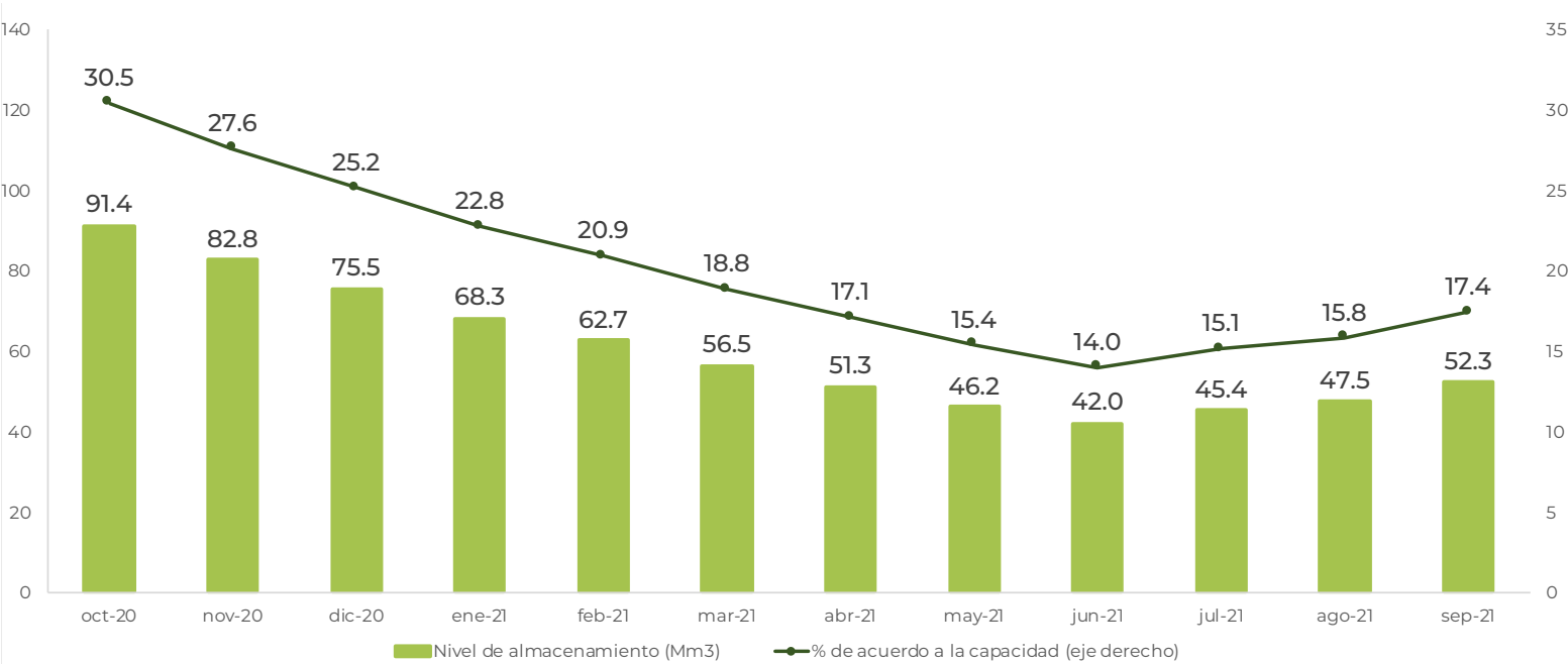
NIVEL DE ALMACENAMIENTO DE AGUA Y PORCENTAJE RESPECTO A LA CAPACIDAD DE LA PRESA CERRO PRIETO octubre 2020 - septiembre 2021
